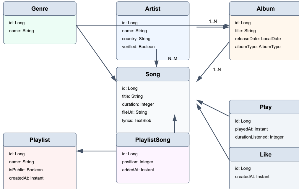
Figura 3. Diagrama de clases simplificado del dominio. Fuente: elaboración propia.
